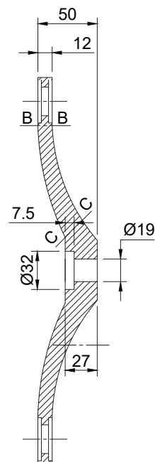
SECTION A-A
