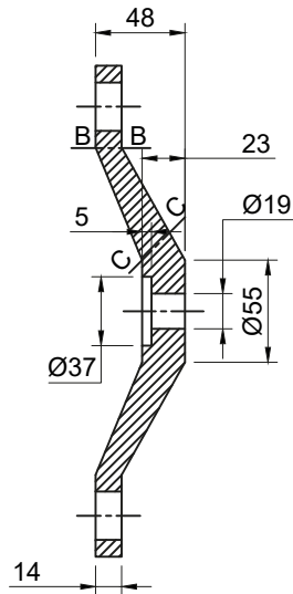
SECTION A-A
